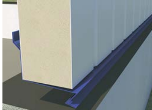
Pieza 1. Elemento que soporta la lámina del remate que va al interior del panel.
