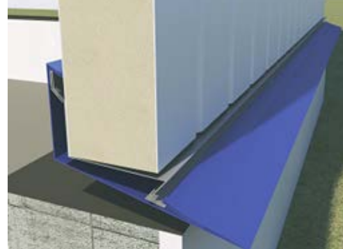
Pieza 2. Elemento que hace clic con la pieza 1, oculta las fijaciones de la pieza 1 y evacua hacia el exterior el agua que pudiera filtrarse.
