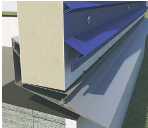
Pieza 3. Elemento anclado a la parte exterior del panel y es encargado de soportar la pieza 4.
